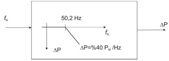
Şekil 7: Frekans yükselmesinde aktif gücün düşmesi
