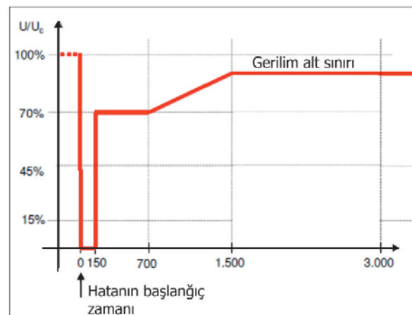
Şekil 5: Birinci tip generatörlerin gerilim eğrisi
